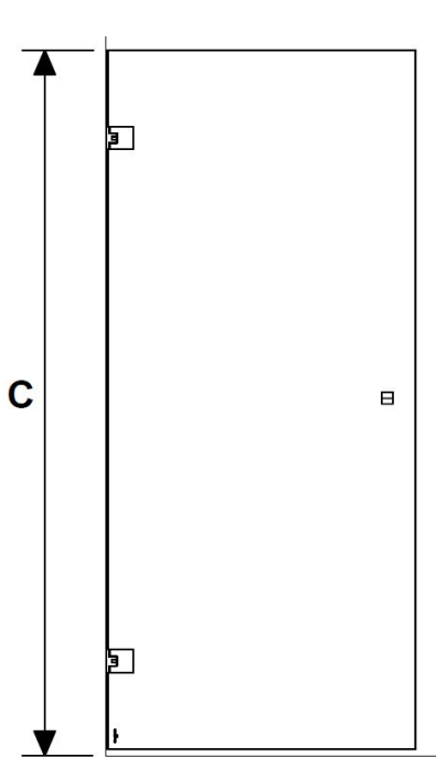
Suihkukulma 1 ovella
